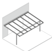
Ü1 Sparrenüberstand, Pfosten außen
